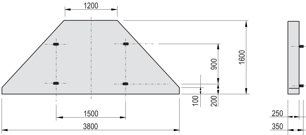
Zentralballaststein ZB 2,5, Art.-Nr.: 30021891
